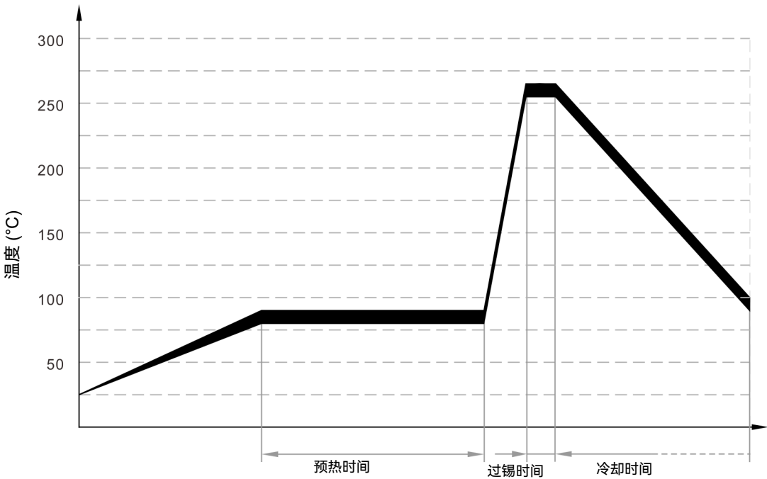
波峰焊曲线
